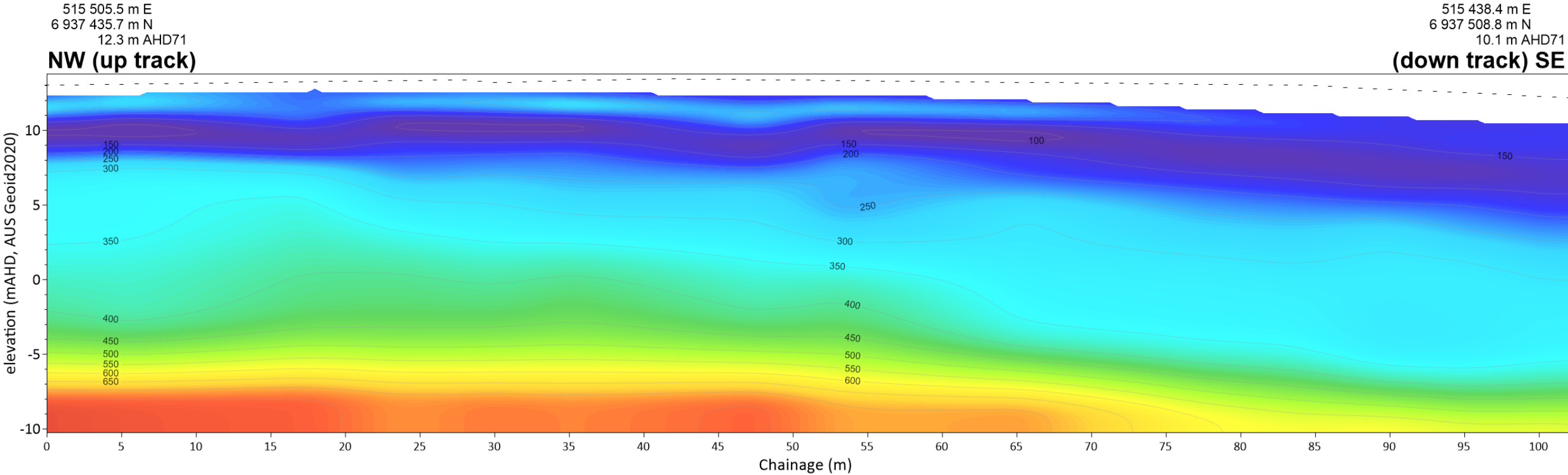
Seismic Line MASW AU-GP 165-1
